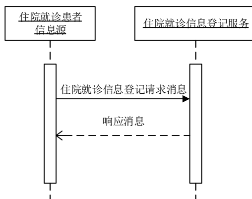
图 14 住院就诊信息登记服务交易流程图
